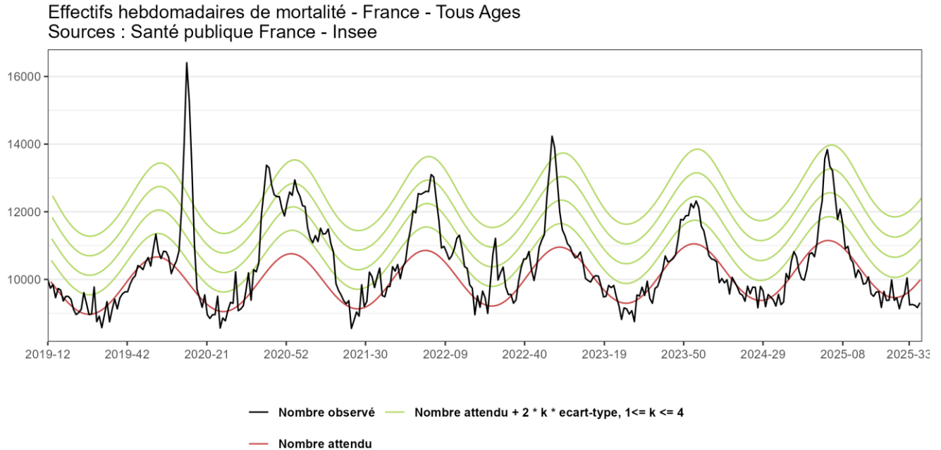
Figure 1 : Fluctuations hebdomadaires des nombres observés (noir) et attendus (rouge) de décès, Tous âges confondus, 2018 à 2024 (jusqu'en semaine 38) - France (Source des données : Insee, actualisation au mardi 30 sept. 2025) (dernière semaine incomplète)
