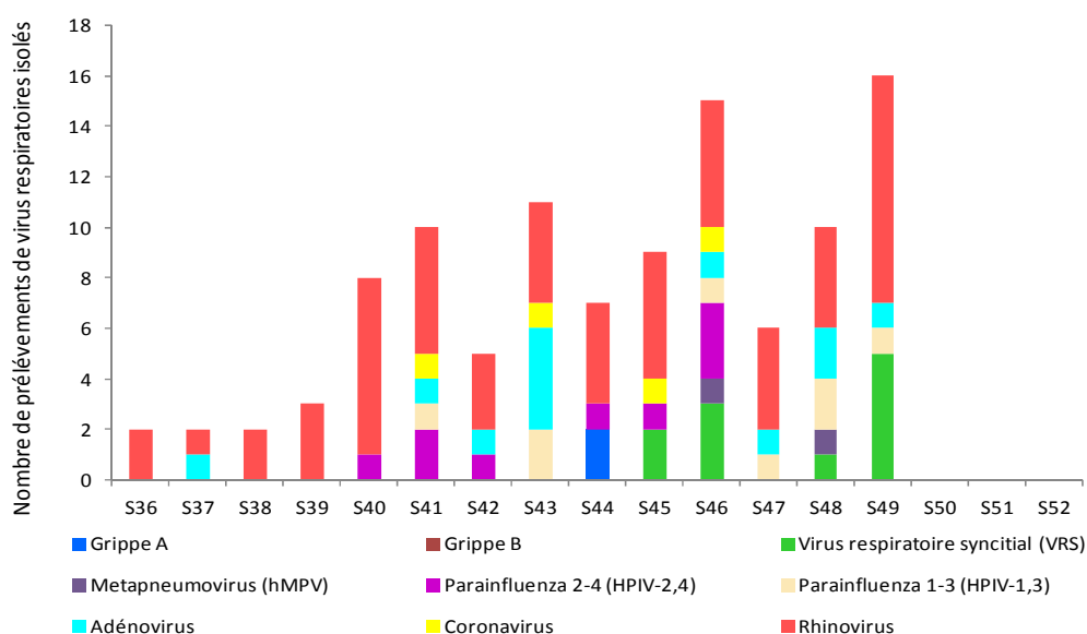
Figure 6 - Evolution hebdomadaire du nombre de prélèvements de virus respiratoires isolés depuis S36-2013
