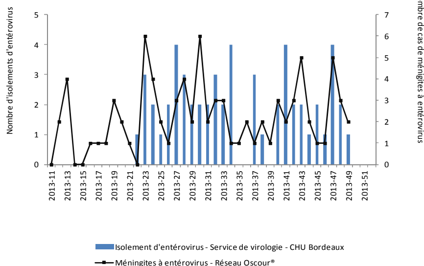
Figure 7 - Evolution hebdomadaire du nb de méningites à entérovirus et des isolations d'entérovirus depuis S11-2013
